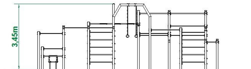
Widok z boku – główne wymiary urządzenia
