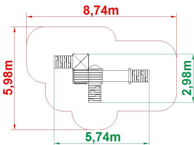
Widok z góry urządzenia
