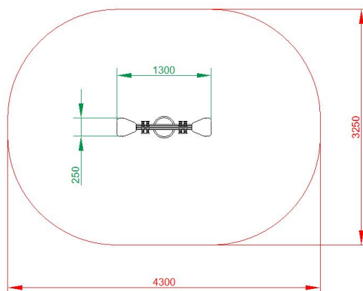
Widok z góry – rozmiar powierzchni zderzenia
