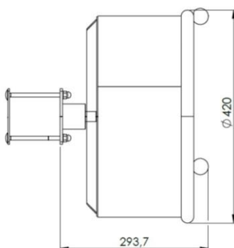
Widok z góry – główne wymiary urządzenia
