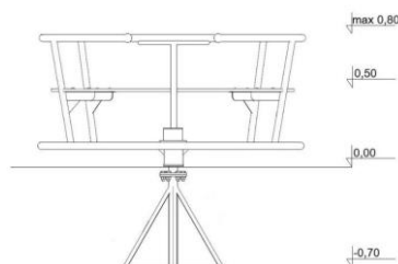
Widok z boku – główne wymiary urządzenia
