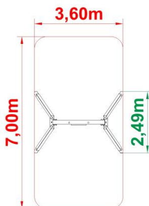
Widok z góry – główne wymiary urządzenia i rozmiar powierzchni zderzenia
