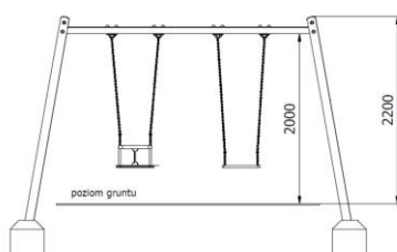
Widok z boku – główne wymiary urządzenia
